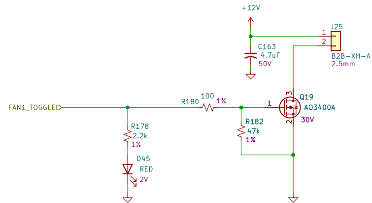
Fan 1
