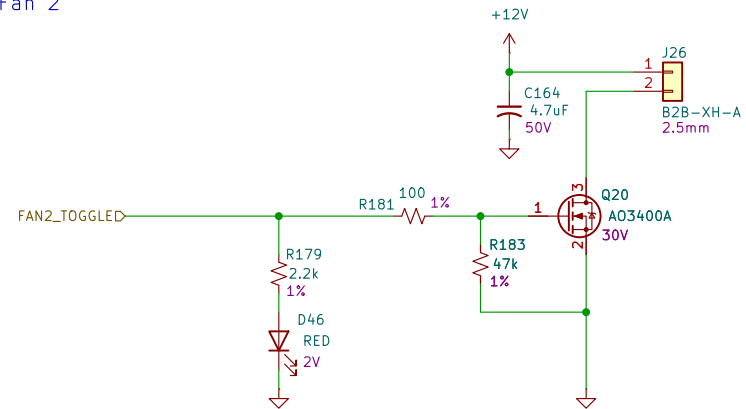
Fan 2
